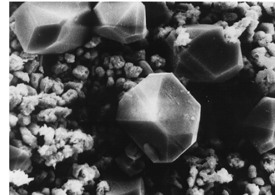
\text{PbSO}_4
